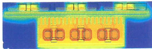
Temperaturprofil eines Fluidgekühlten Mittelspannungsumrichters
