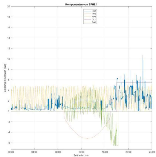
Abbildung 34: Gebäude EFH8.1 in der Topologie Dorf 1 mit Eingriff, links Gesamtlastgang, rechts einzelne Bestandteile des Lastganges
