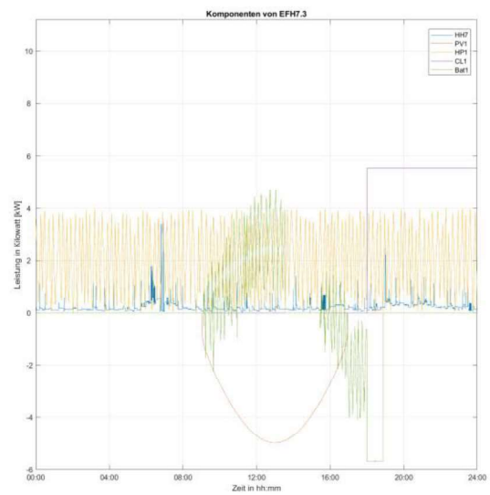
Abbildung 32: Gebäude EFH7.3 in der Topologie Dorf 1 mit Eingriff, links Gesamtlastgang, rechts einzelne Bestandteile des Lastganges
