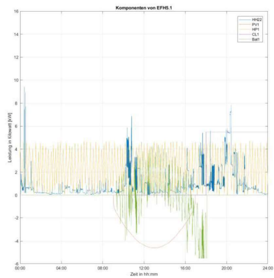
Abbildung 24: Gebäude EFH5.1 in der Topologie Dorf 1 mit Eingriff, links Gesamtlastgang, rechts einzelne Bestandteile des Lastganges
