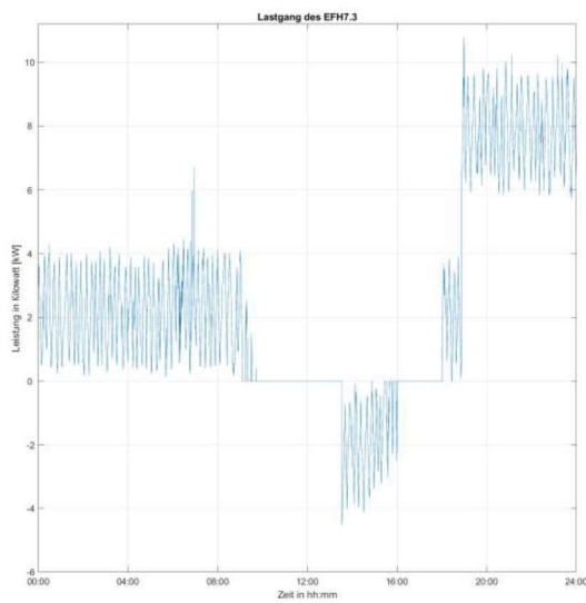
Abbildung 32: Gebäude EFH7.3 in der Topologie Dorf 1 mit Eingriff, links Gesamtlastgang, rechts einzelne Bestandteile des Lastganges
