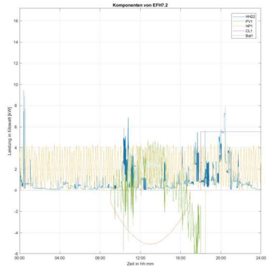
Abbildung 31: Gebäude EFH7.2 in der Topologie Dorf 1 mit Eingriff, links Gesamtlastgang, rechts einzelne Bestandteile des Lastganges
