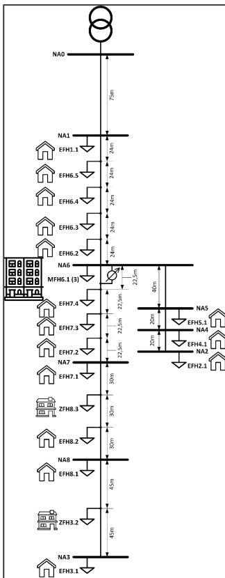
Abbildung 54: Topologie Dorf 1.
