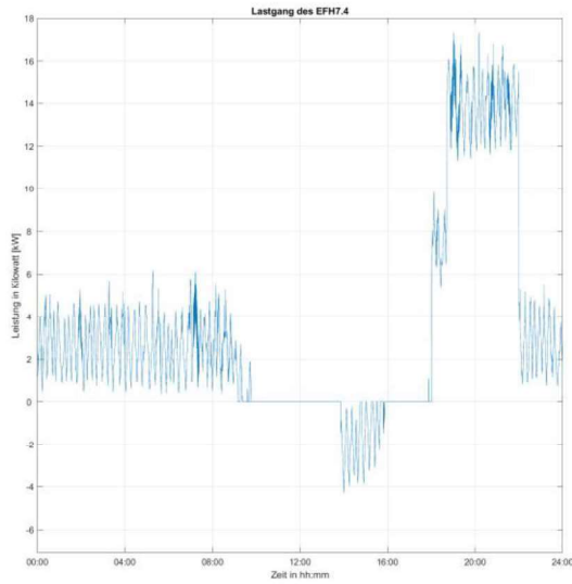
Abbildung 15: Gebäude EFH7.4 in der Topologie Dorf 1, links Gesamtlastgang, rechts einzelne Bestandteile des Lastganges
