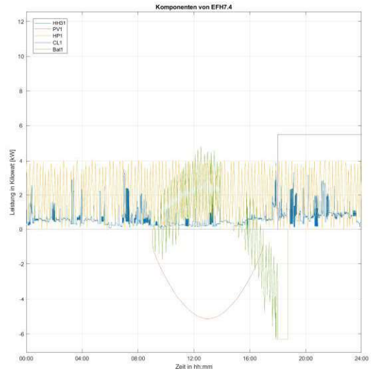
Abbildung 33: Gebäude EFH7.4 in der Topologie Dorf 1 mit Eingriff, links Gesamtlastgang, rechts einzelne Bestandteile des Lastganges
