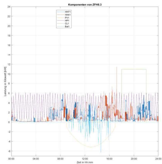
Abbildung 18: Gebäude ZFH8.3 in der Topologie Dorf 1, links Gesamtlastgang, rechts einzelne Bestandteile des Lastganges
