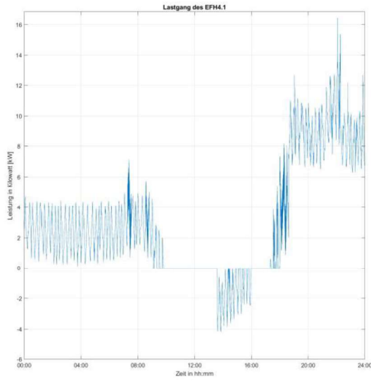
Abbildung 23: Gebäude EFH4.1 in der Topologie Dorf 1 mit Eingriff, links Gesamtlastgang, rechts einzelne Bestandteile des Lastganges
