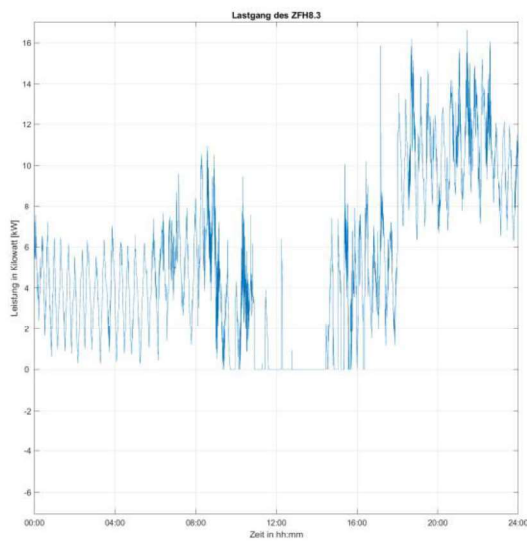
Abbildung 36: Gebäude ZFH8.3 in der Topologie Dorf 1 mit Eingriff, links Gesamtlastgang, rechts einzelne Bestandteile des Lastganges
