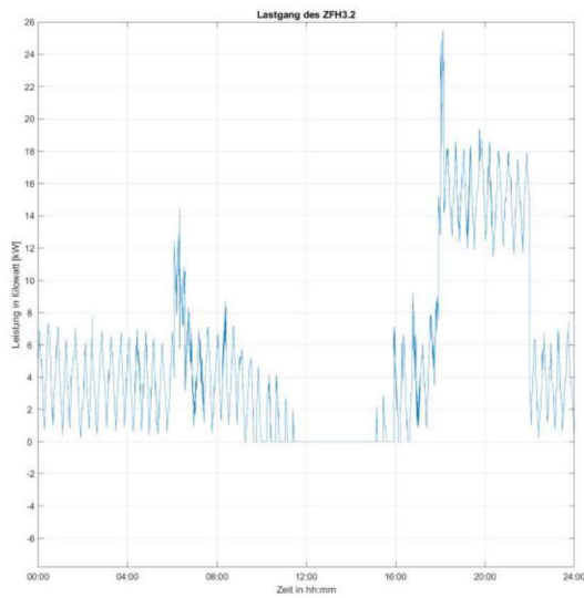
Abbildung 4: Gebäude ZFH3.2 in der Topologie Dorf 1, links Gesamtlastgang, rechts einzelne Bestandteile des Lastganges
