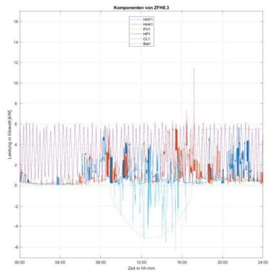
Abbildung 36: Gebäude ZFH8.3 in der Topologie Dorf 1 mit Eingriff, links Gesamtlastgang, rechts einzelne Bestandteile des Lastganges
